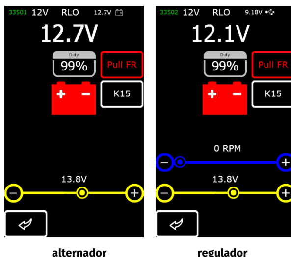
Figura 12. Pantalla del diagnóstico del alternador/regulador del tipo RLO, RVC, C KOREA
