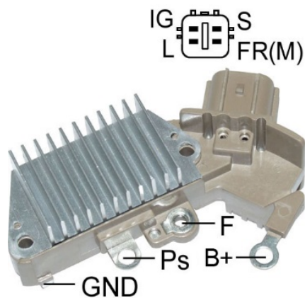
Figura 21. Regulador ARE6076
