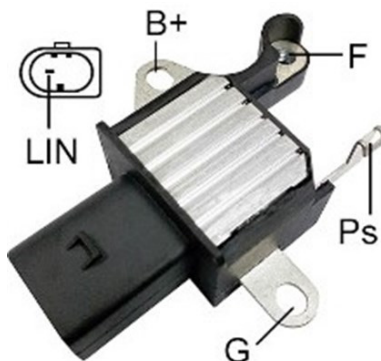
Figura 23. Regulador ARE6149P
