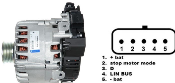
Figura 25. Alternador Valeo IST60C017 y designación de terminales en el conector
