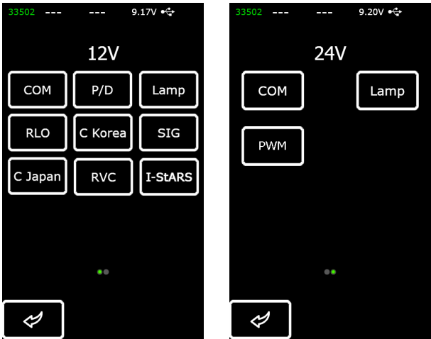
Figura 9. Menú de selección del tipo de alternador/regulador a diagnosticar
