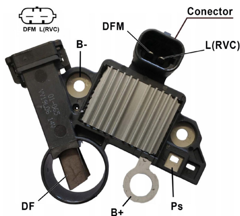
Figura 19. Regulador ARE1054
