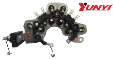
แผงไดโอด HINO MEGA 500 12340100 2-371-33-05
