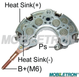
แผงไดโอด Toyota 80A อลู หลักลม 103mm M6 RN-03PL 2-374-01-02
