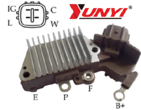
คัทเออร์ท HINO MEGA500 ปลั๊กเต้านอน 24V 1332DZ00 2-066-04-14
