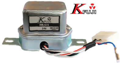
คัทเออร์ทนอกตัว ระบบอิเล็กทรอนิกส์ IVR-615 24V K.FUJI 2-068-06-01
