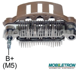
แผงไดโอด Mibiltron RM-181 Honda Civic FD Mitsu 8เม็ต 85mm M5 2-374-01-03
